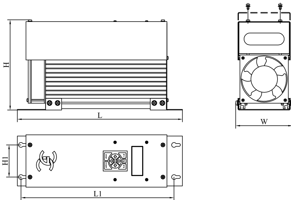
Рис. 9 Габаритные и установочные размеры контроллера ЭнерджиСейвер ES11-45
