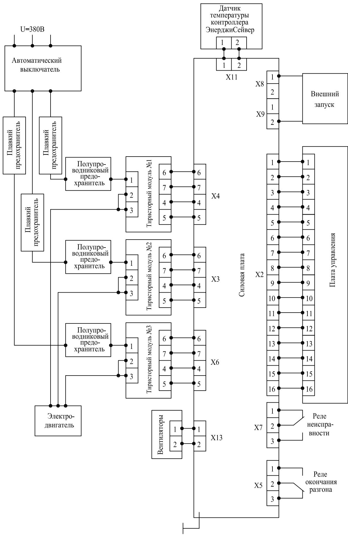
Рис. 5 Общая схема подключения контроллера ЭнерджиСейвер (ES55-ES200)
