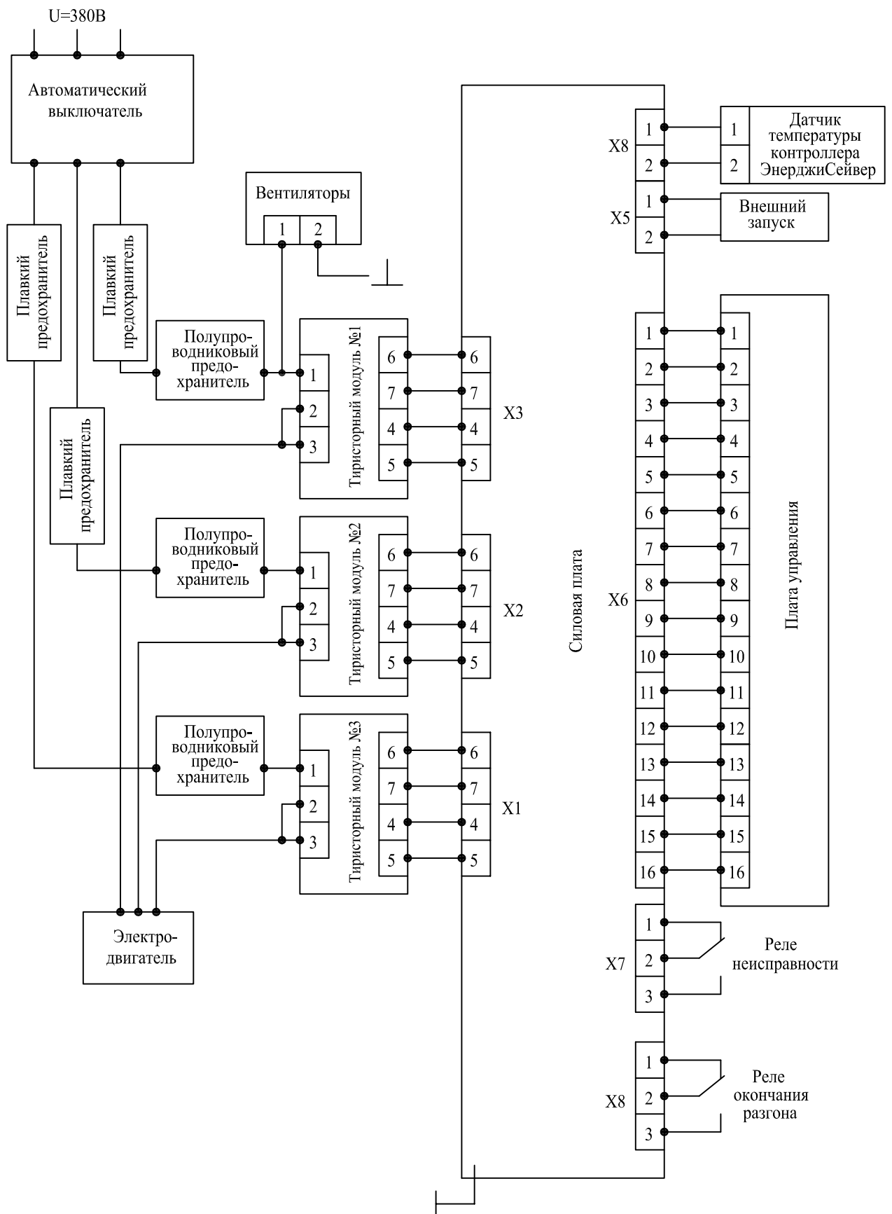
Рис. 4 Общая схема подключения контроллера ЭнерджиСейвер (ES11-ES45)
