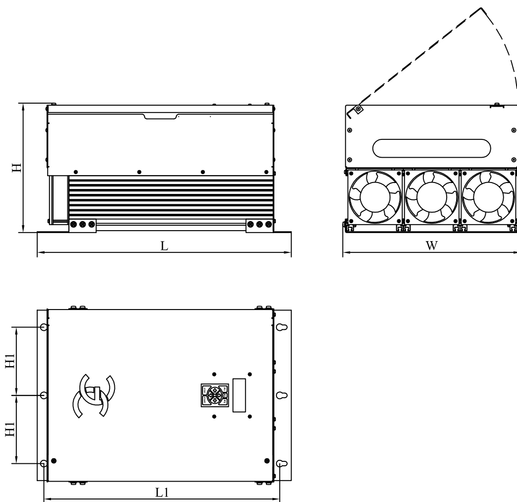
Рис. 10 Габаритные и установочные размеры контроллера ЭнерджиСейвер ES55-200
