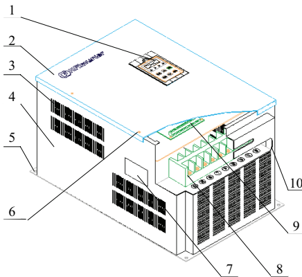
Рис 2-4 Металлический корпус
