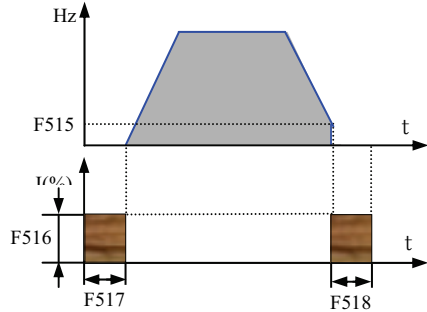
Fig 5-9 Торможение
