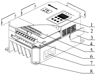
Рис 2-3 Пластмассовый корпус
