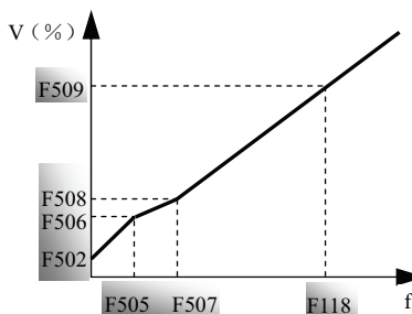
Рис 5-8 Многоугольная V/F
